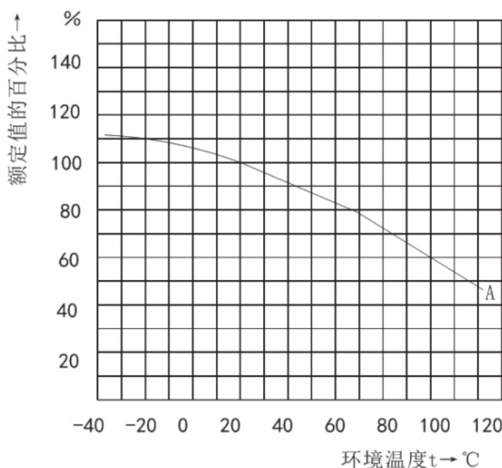
环境温度对电流承载能力影响的典型曲线
